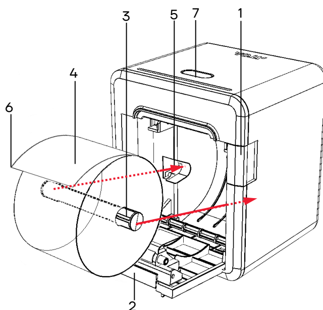
Рисунок 11. Заправка бумаги при вертикальной установке ККТ
