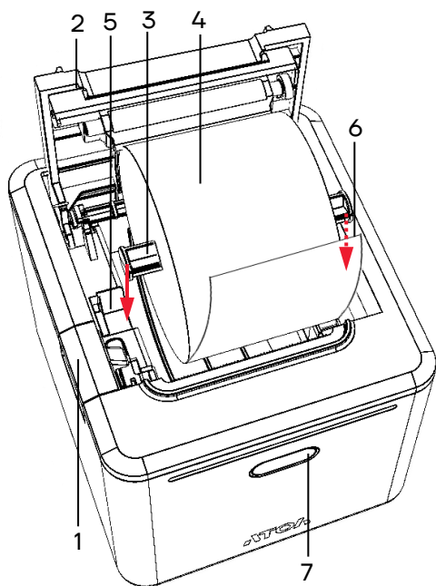
Рисунок 10. Заправка бумаги при горизонтальной установке ККТ
