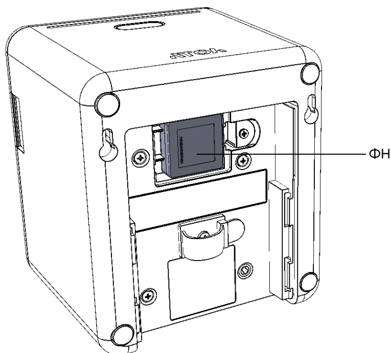
Рисунок 5. Место расположения ФН в корпусе ККТ (крышка отсека ФН и крышка разъемов условно не показаны)
