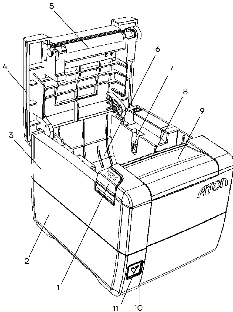
Рисунок 1. Внешний вид ККТ
