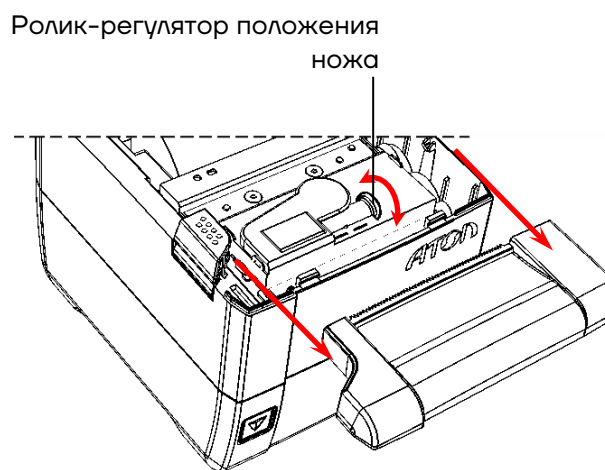
Рисунок 7. Ролик-регулятор положения ножа автоотрезчика
