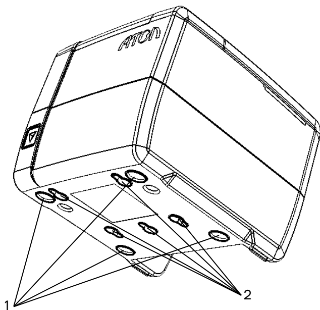
Рисунок 4. Вертикальное крепление ККТ
