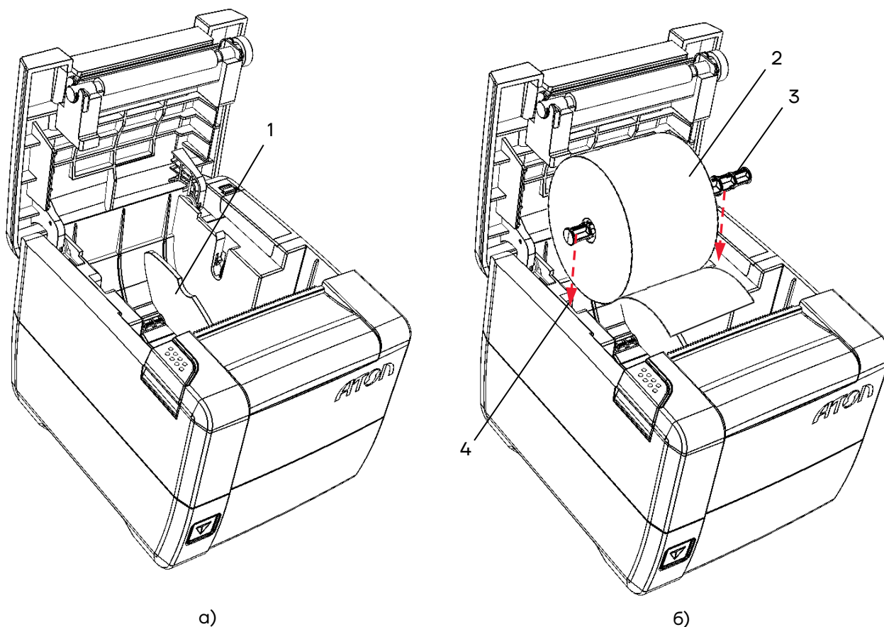
Рисунок 6. Установка ЧЛ 58 мм: а) установить ограничитель; б) установить ось с рулоном ЧЛ в пазы лотка для ЧЛ
